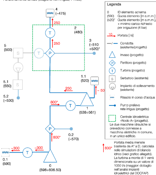
Diga di Casalbuono - Schema idrico - Alternativa 2 Funzionamento invernale (stagione non irrigua, 7 mesi)
