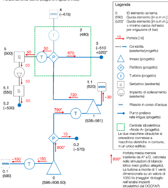
Diga di Casalbuono - Schema idrico - Alternativa 2 Funzionamento estivo (stagione irrigua, 5 mesi)
